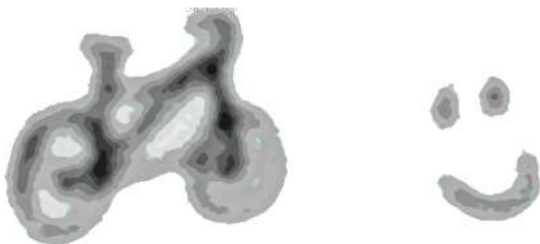
Figure 1: Sketch of the CNO bi-cycle (Ödman, 2004).
